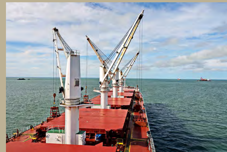
デッキクレーン Deck Crane
